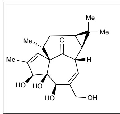
(+)-Ingenol
