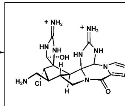
Palau'amine
